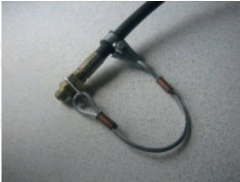
Abbildung 17: Seilverbindung
